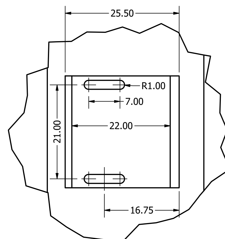
DETALLE G
