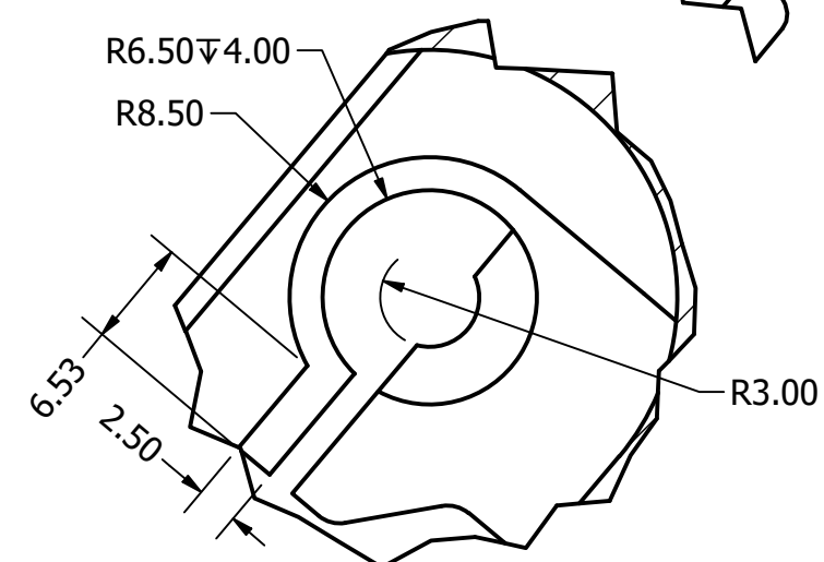
DETALLE E
